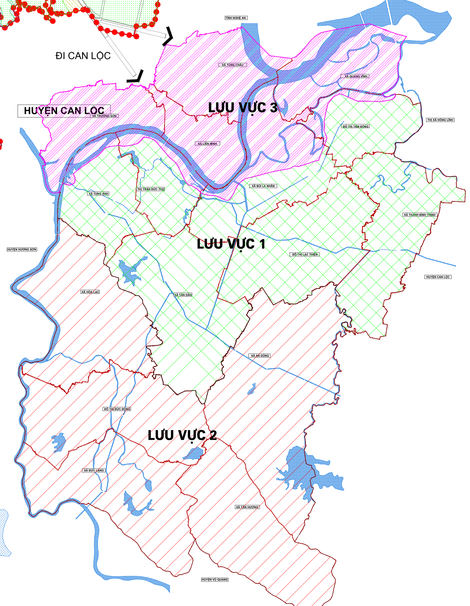
SƠ ĐỒ DỰ KIẾN PHÂN LƯU VỰC THOÁT NƯỚC CHÍNH
